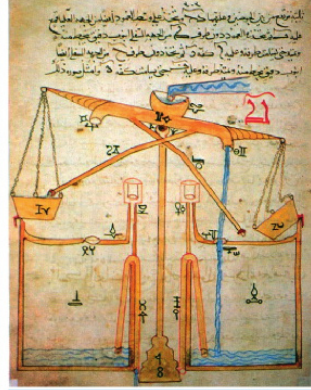
El-Cezeri'nin icat ettiği iki şamandıralı fiskeye
